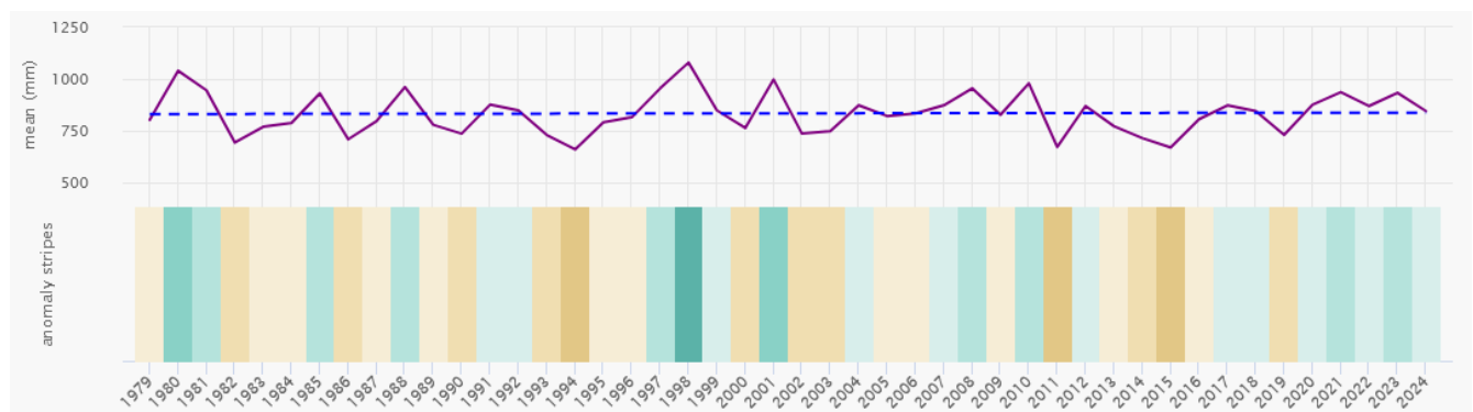
Рис.2.3. Річна зміна опадів у Бібрській МТГ
