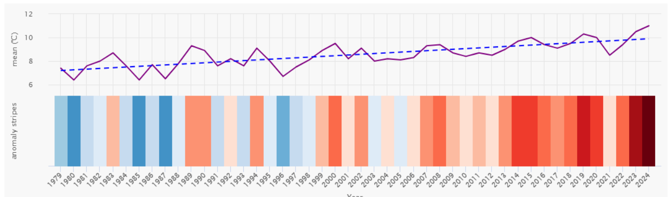
Рис.2.2. Річна зміна температури у Бібрській МТГ
